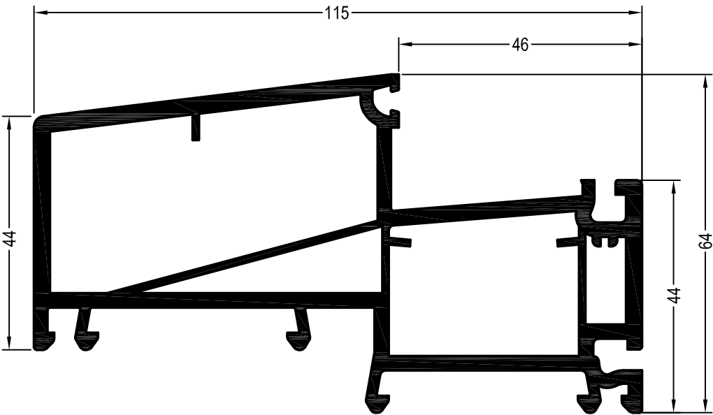
Профили коробок
