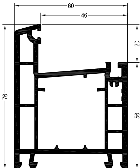
Профили коробок
