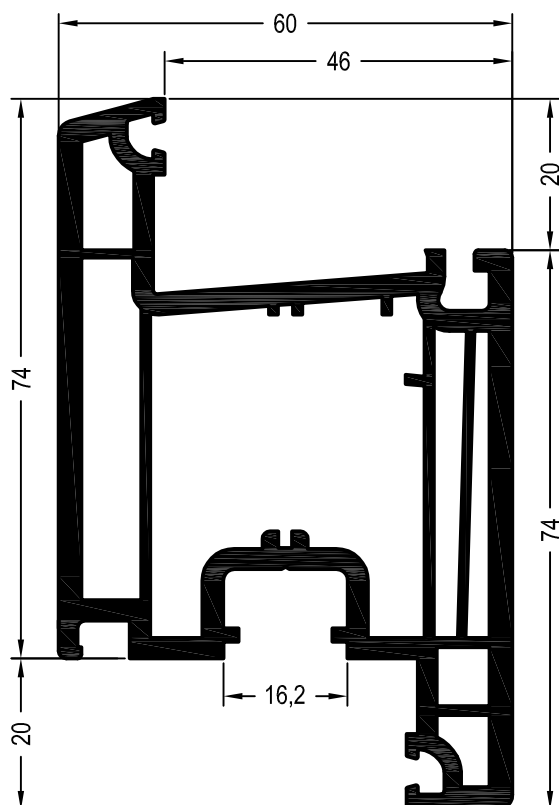
Профили створок
